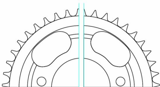
Piñón/Corona correcto
